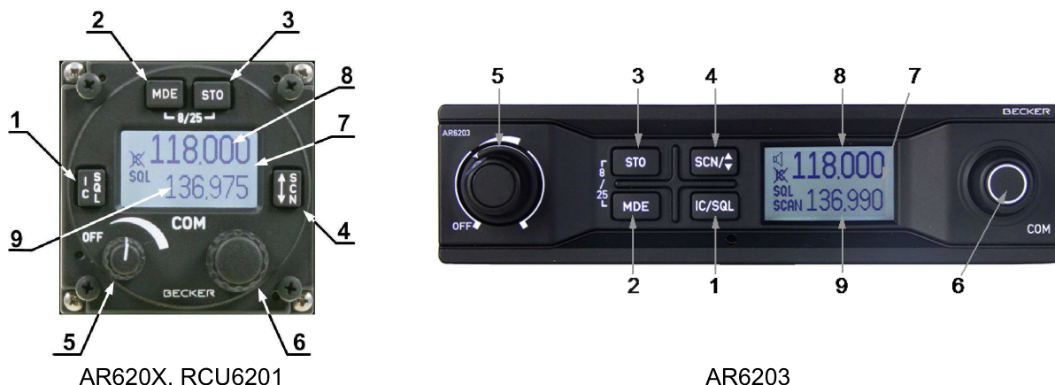
Illustration 3-1 : Commandes et indicateurs
